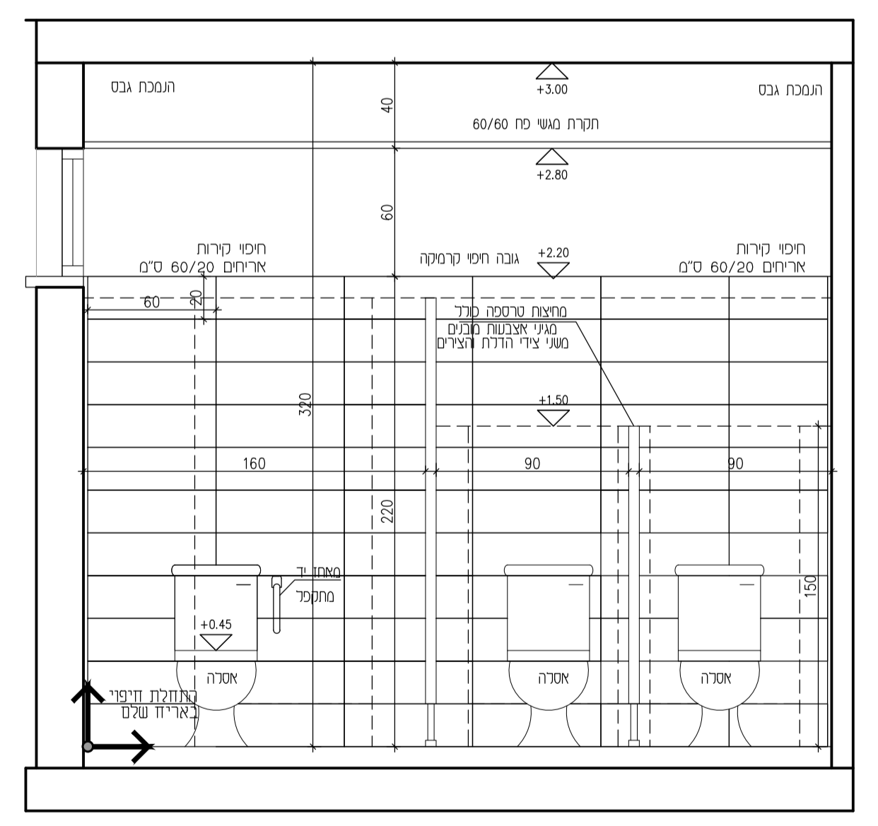
חזית 3
