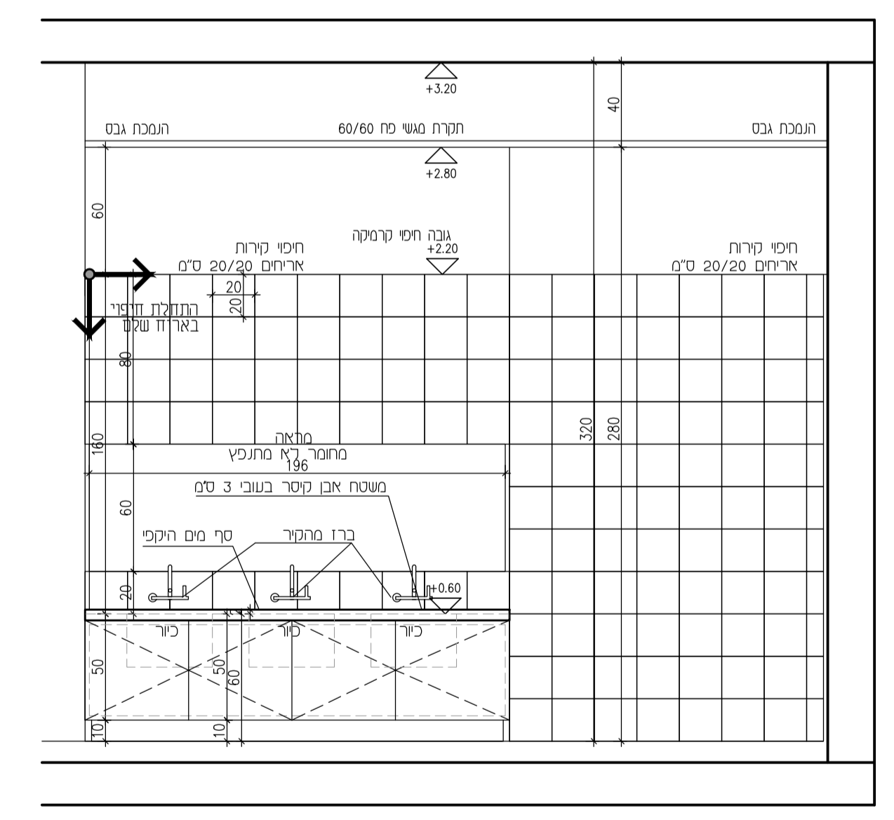
חזית 1
