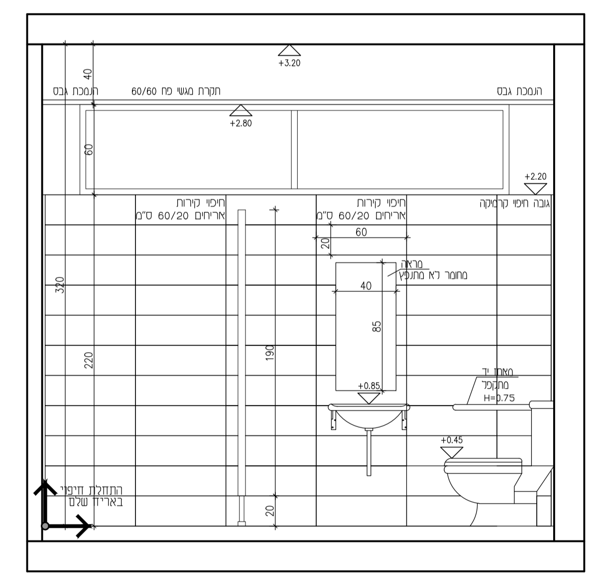
חזית 2
