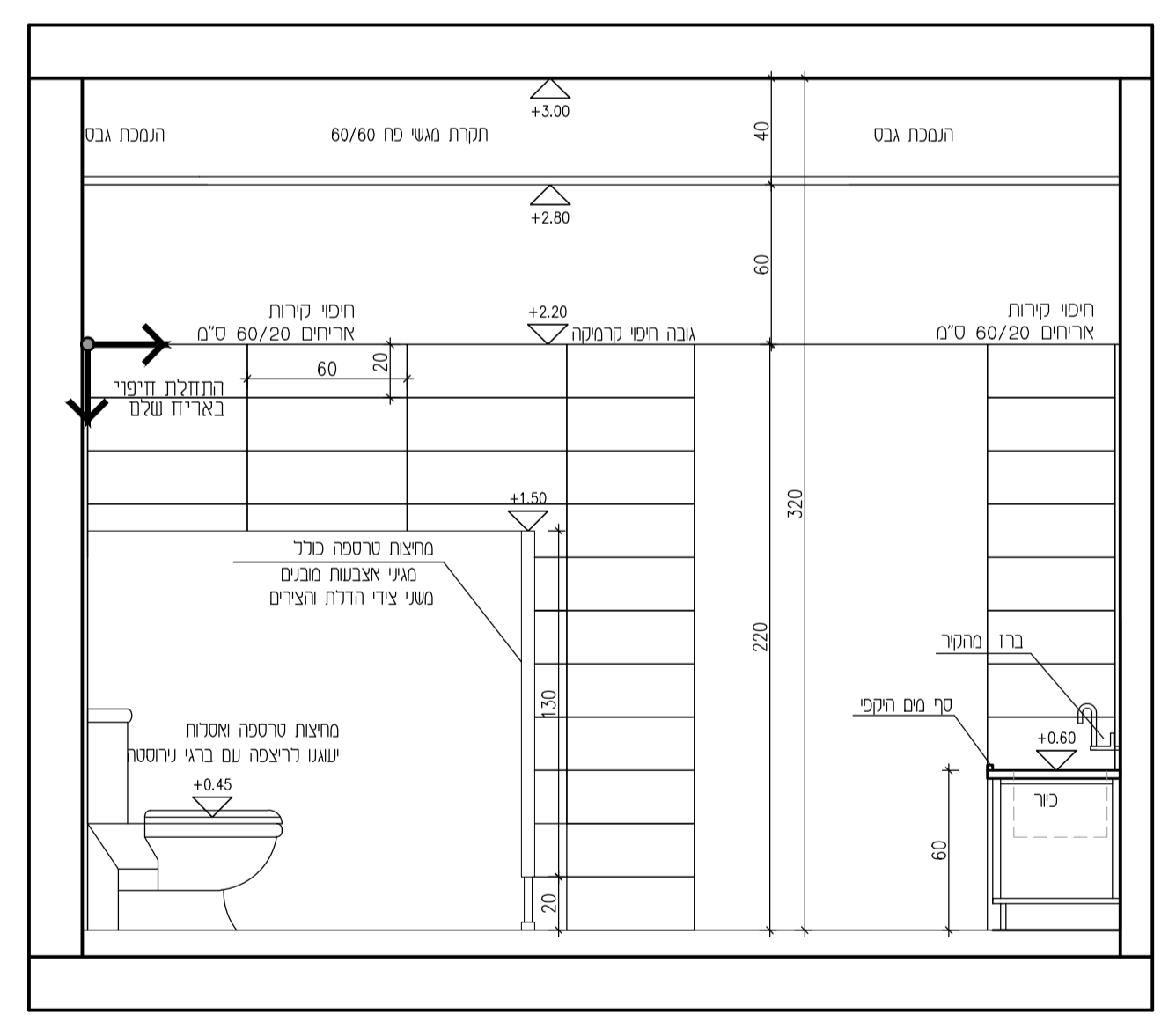
חזית 4
